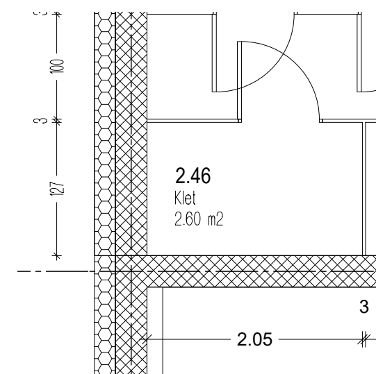
Objekt 2 - 5. nadstropje
